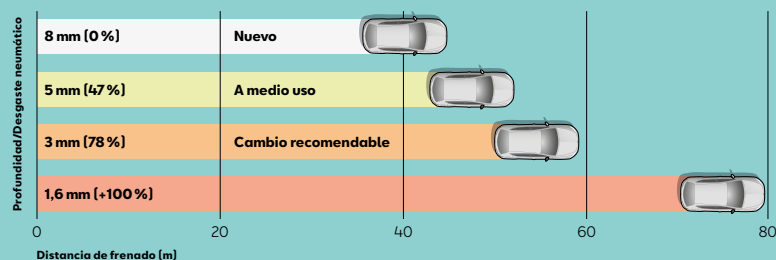
Distancia de frenado (m) de 100 a 60 km/h sobre asfalto mojado.
